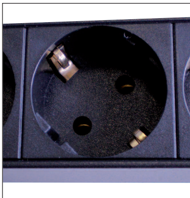
2 Pin DIN49441 Socket
